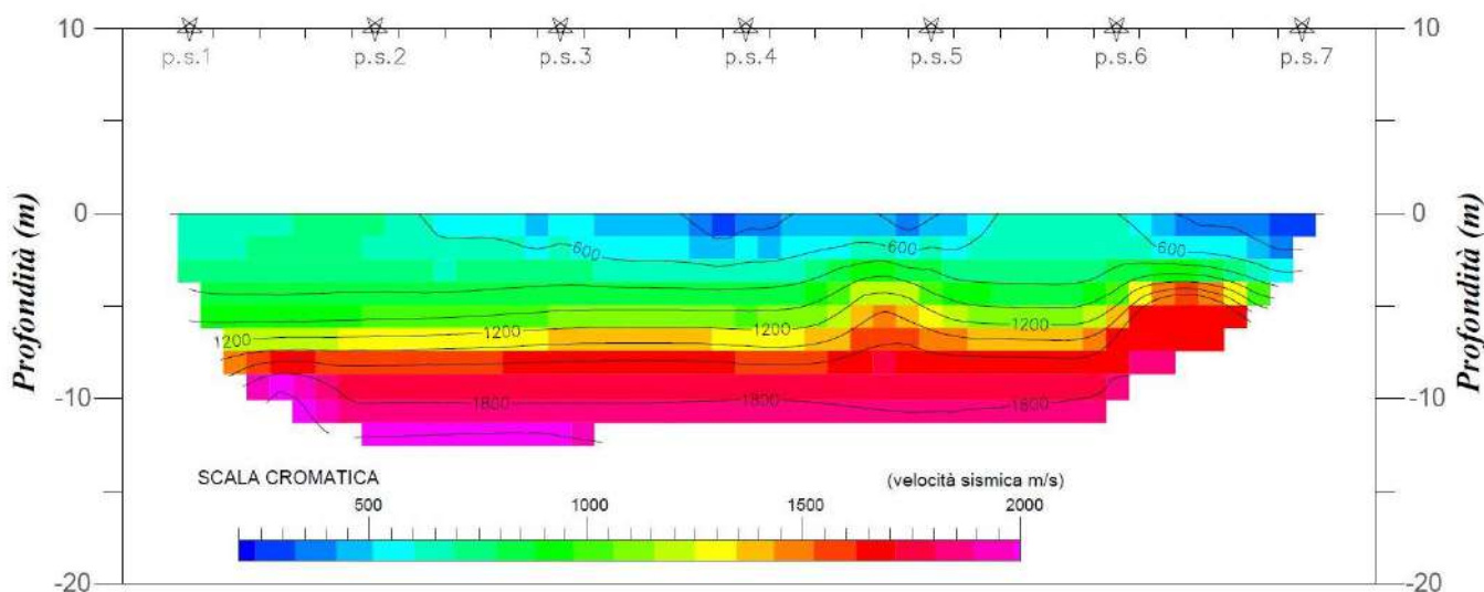
Sezione sismostratigrafica
